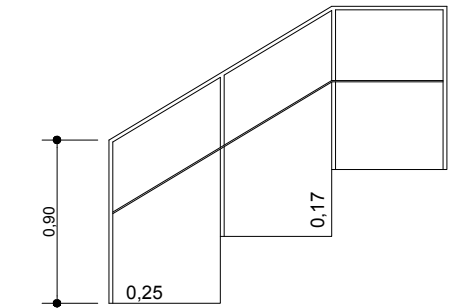
DETALHE GENÉRICO ESCADA SEM ESCALA
