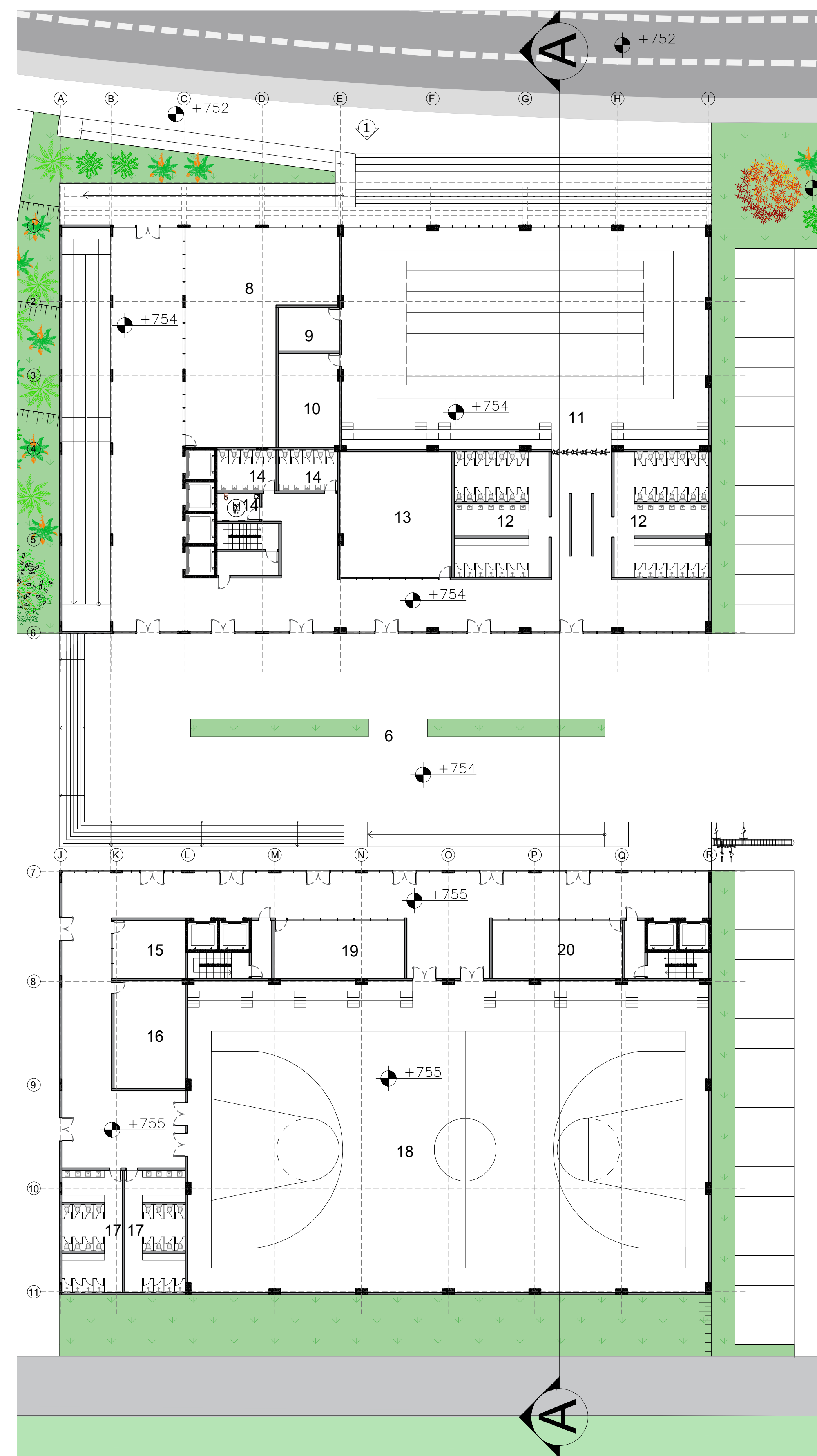
TERREO - EDIFICIO ESCALA: 1/250
