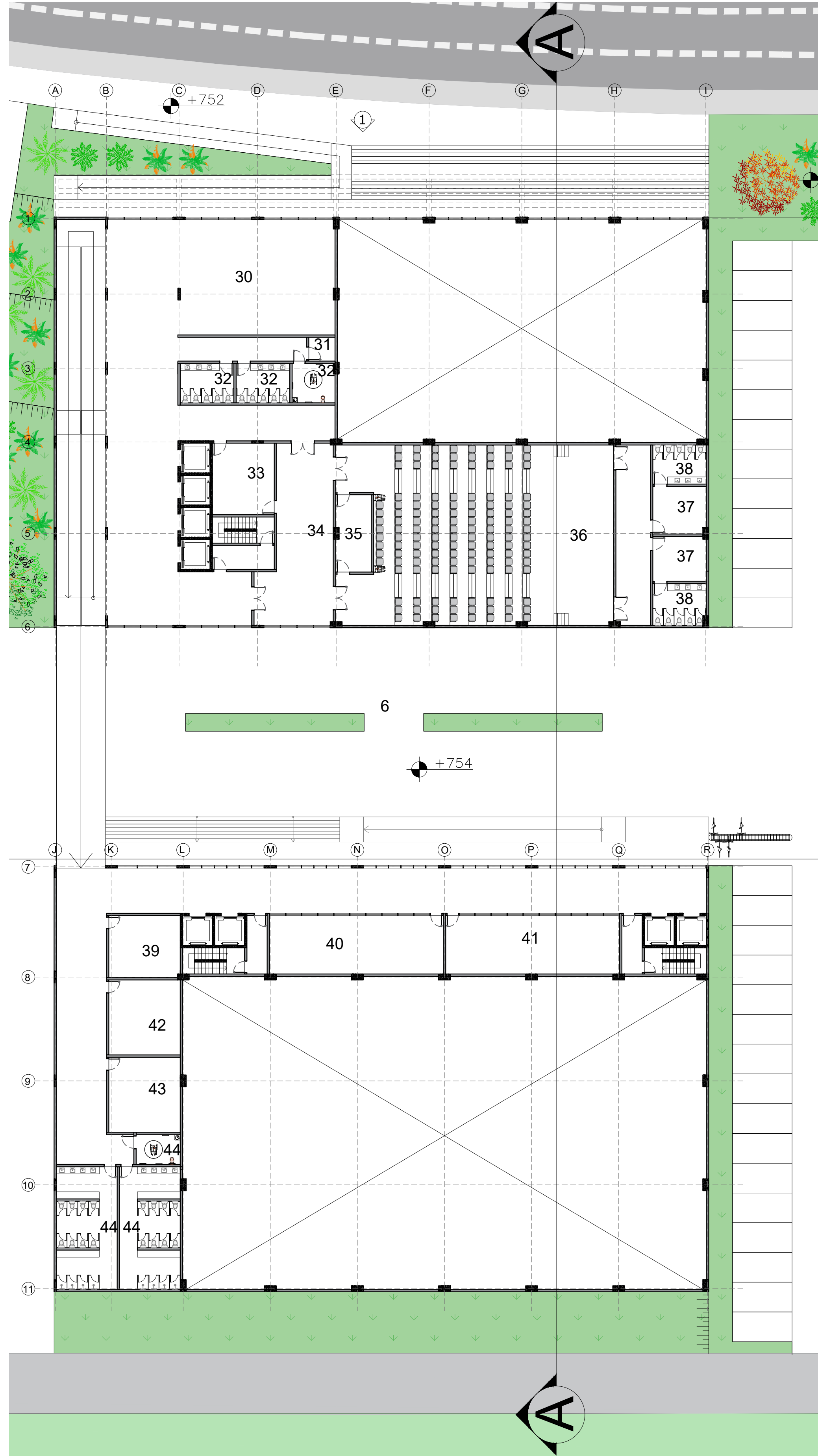
3- PAVIMENTO ESCALA: 1/250
