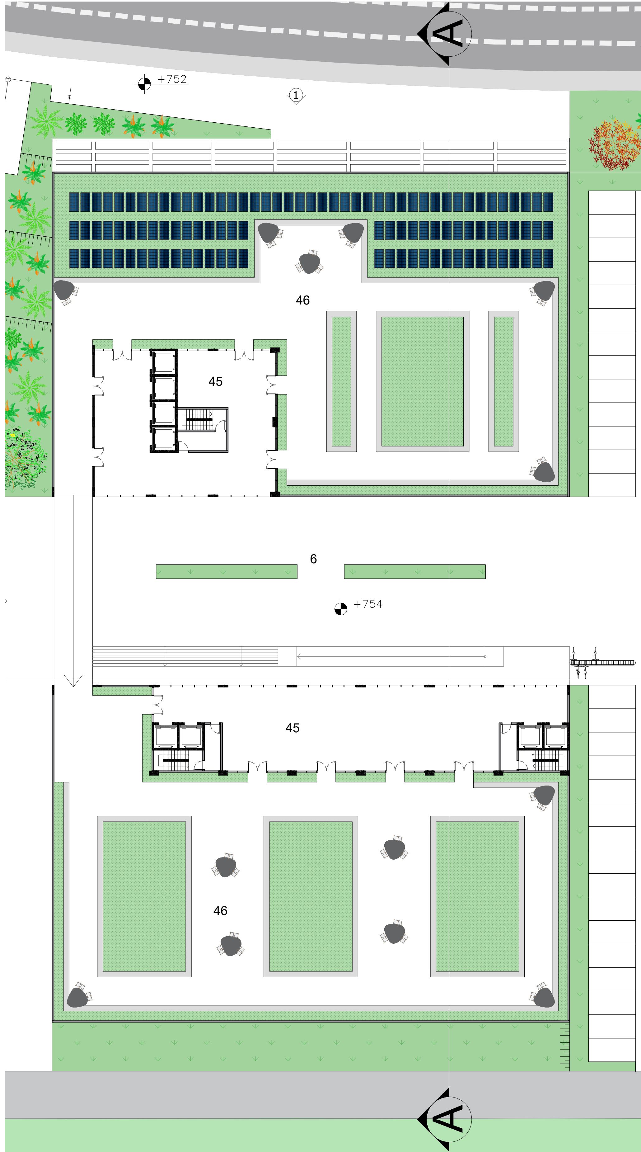
COBERTURA ESCALA: 1/250
