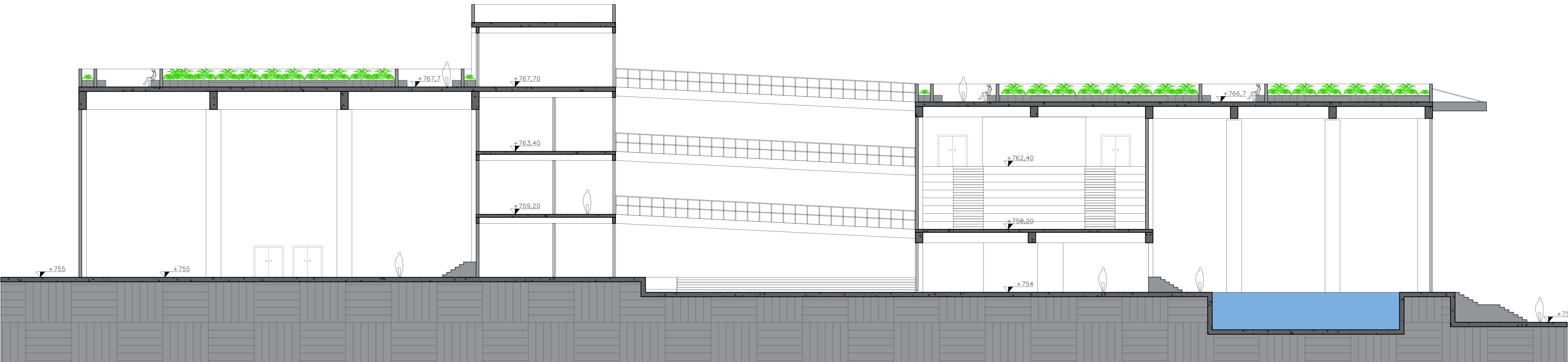
CORTE AA ESCALA: 1/100
