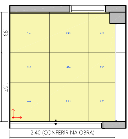
VISTA 01 ESCALA 1:50
