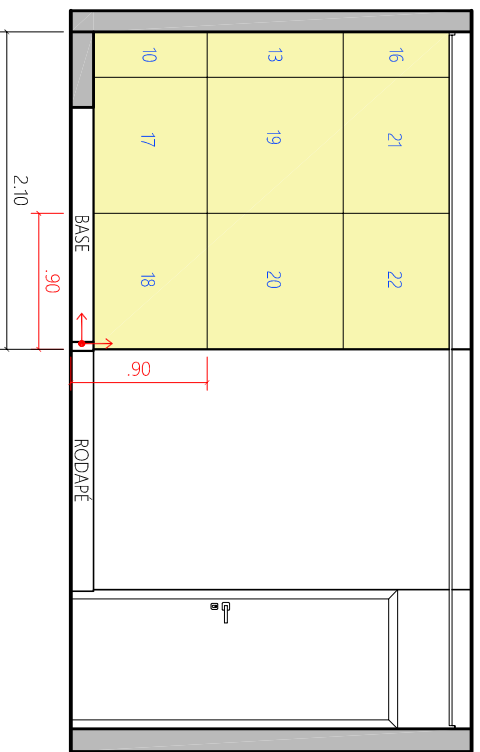
VISTA 03 ESCALA 1:50
