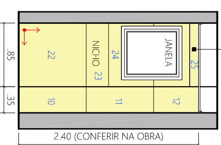
VISTA 04 ESCALA 1:50
