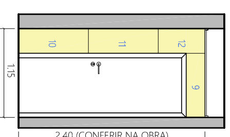
VISTA 02 ESCALA 1:50
